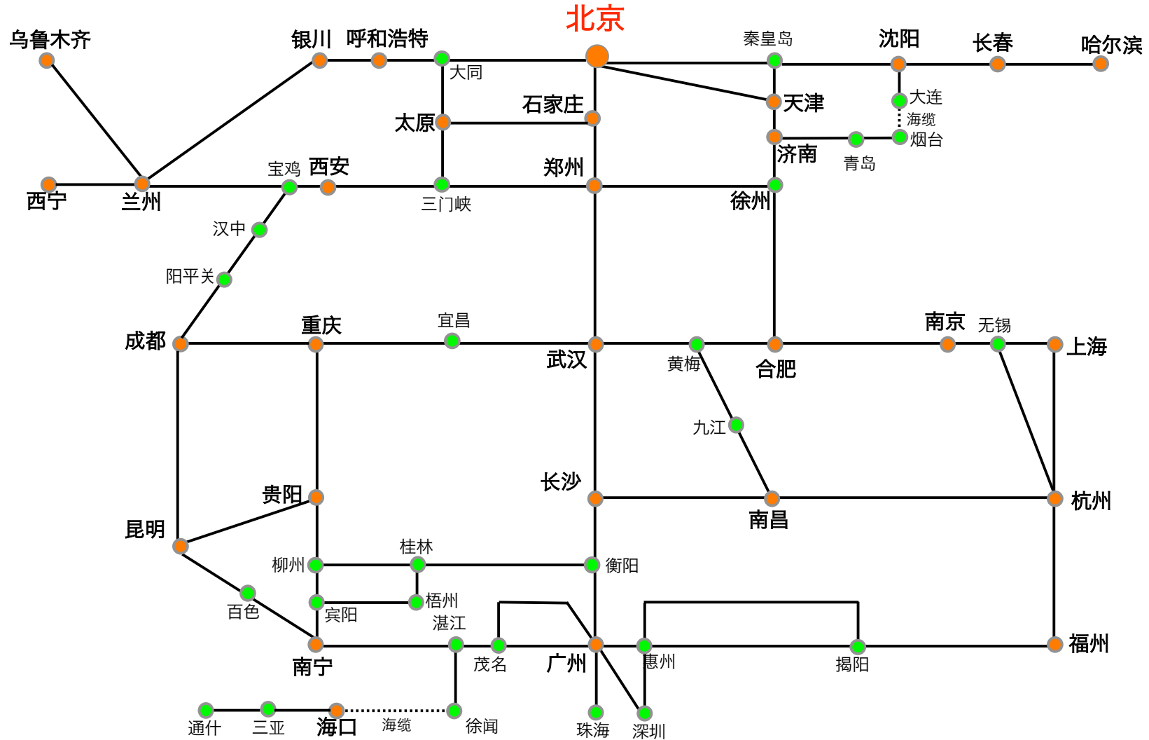
全国光缆干线网络拓扑结构图
